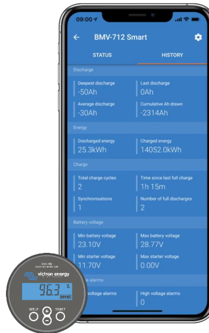
BMV
