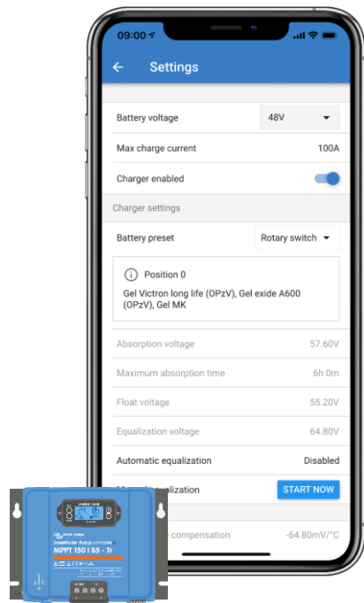
MPPT
